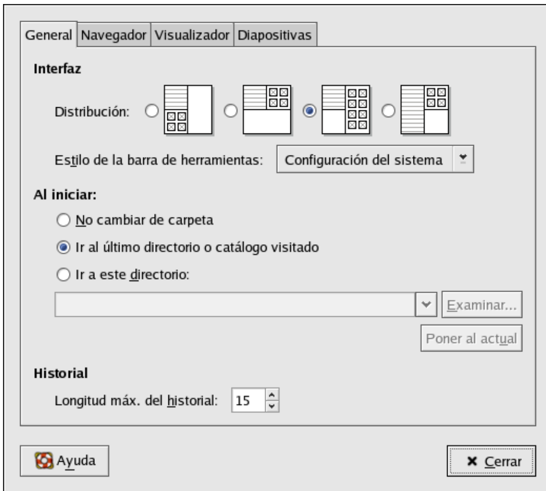
Figura 11-4. La ventana de diálogo de Preferencias de GThumb
