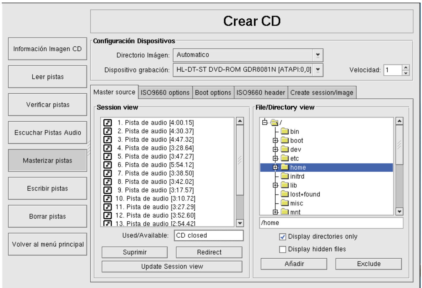
Figura 4-10. Uso de X-CD-Roast para respaldar archivos del disco duro
